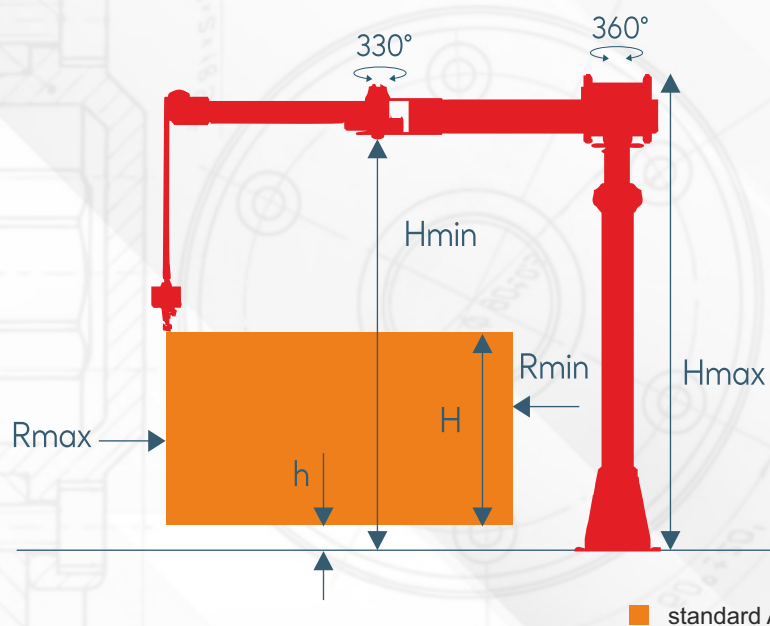
Bodenmontage
