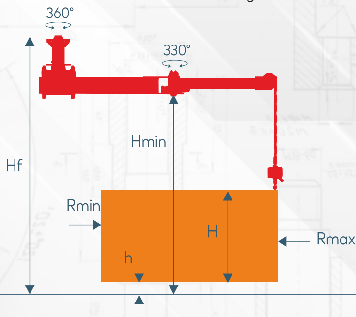
Deckenmontage
