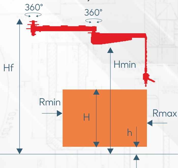
Montaje en techo
