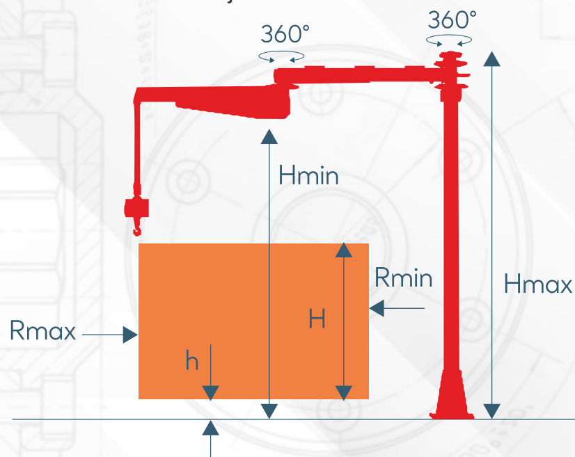
Montaje en el suelo
