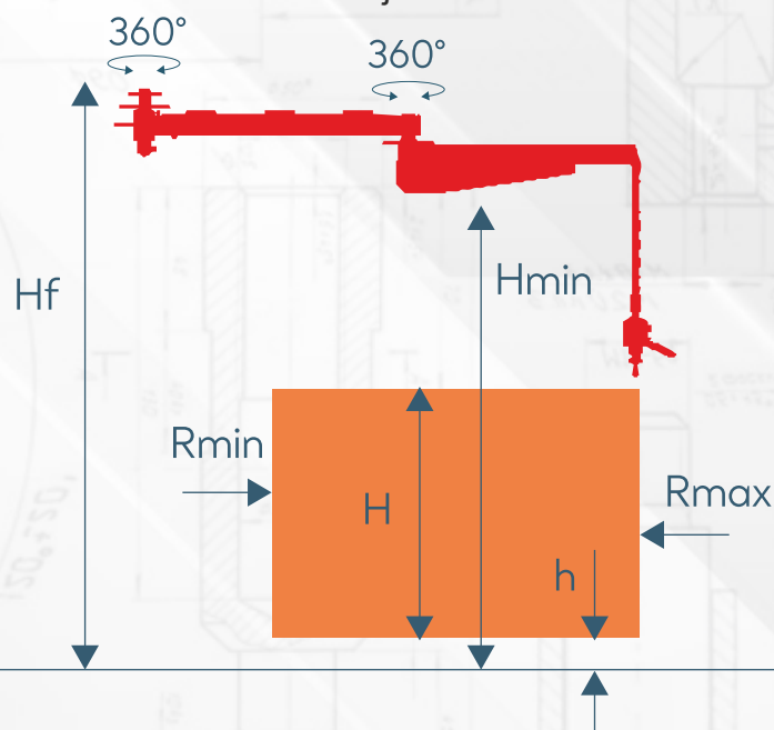
Montaje en techo
